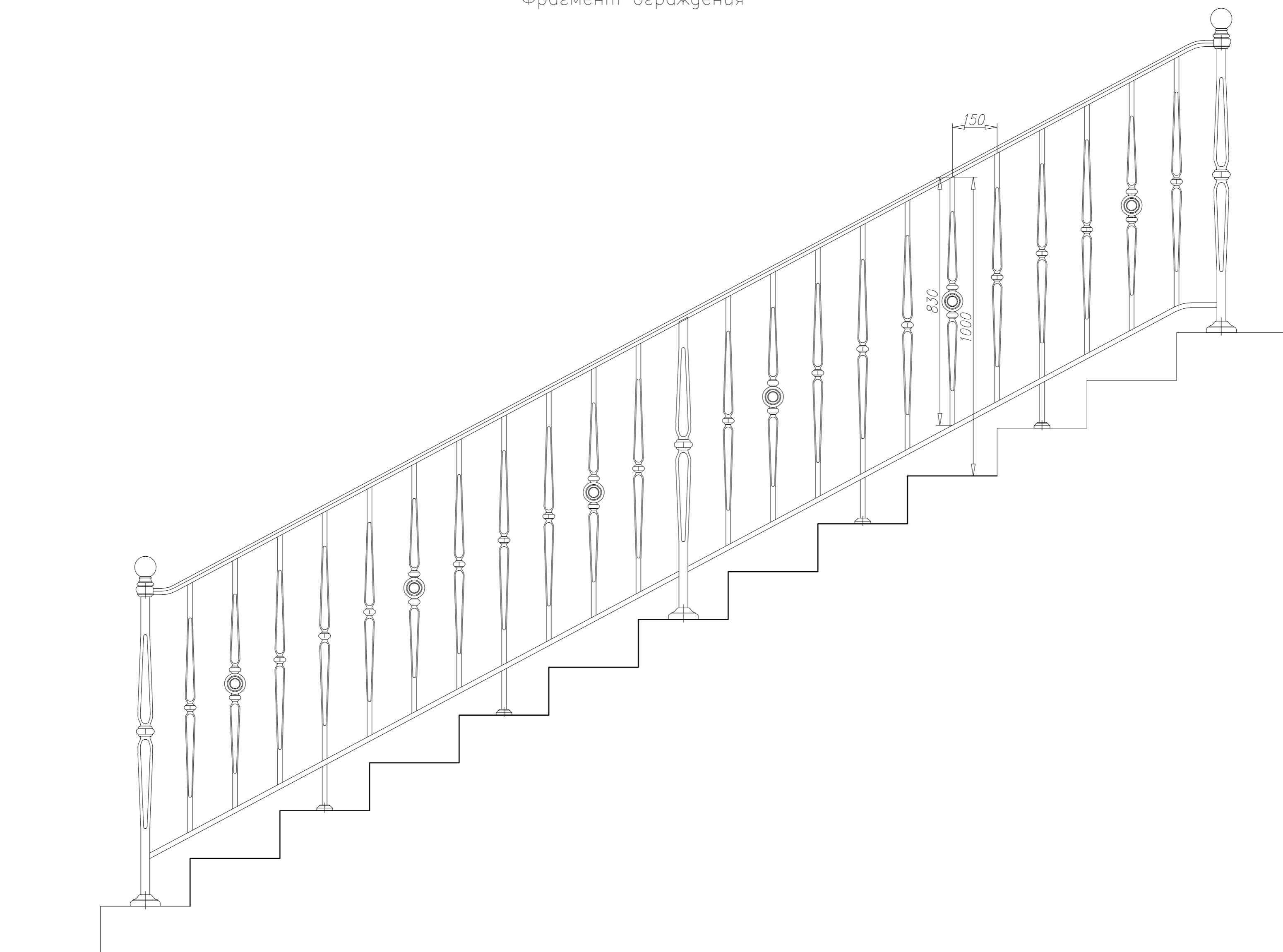
Серия "Рондо" Вариант 1 Фрагмент ограждения
